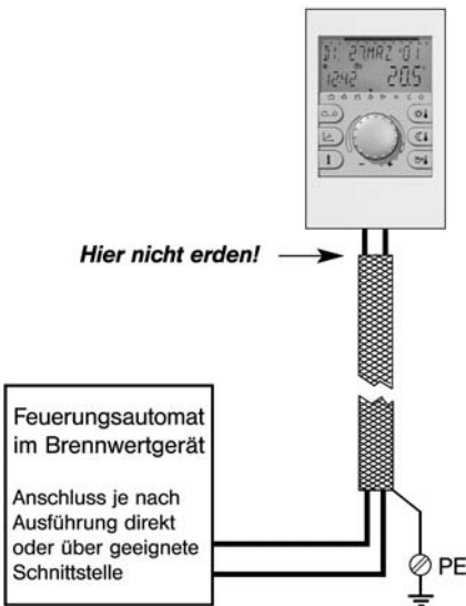
Bild 4: Einseitige Erdung der Abschirmung
