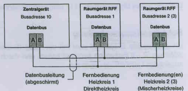
Abb.3 Datenbusführung
